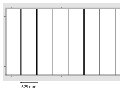
Metallkonstruktion Montageschritt 2
